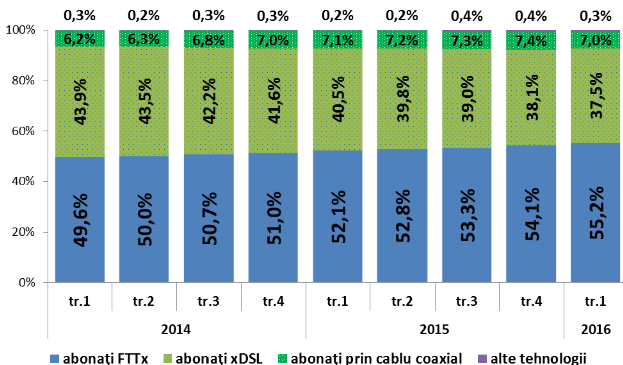
Figura 32. Structura pieței serviciilor în bandă largă în funcție de tehnologia de acces
