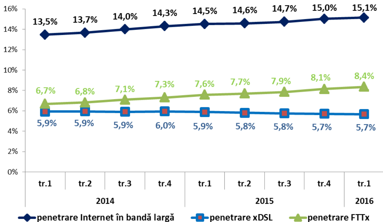
Figura 33. Evoluția ratelor de penetrare
